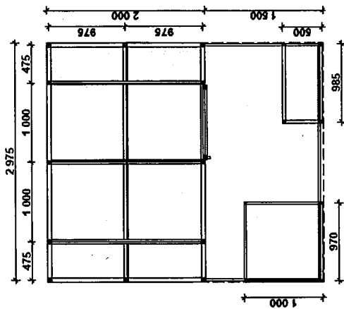
Вид сверху
