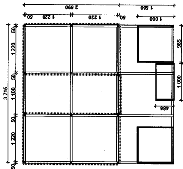
Вид сверху
