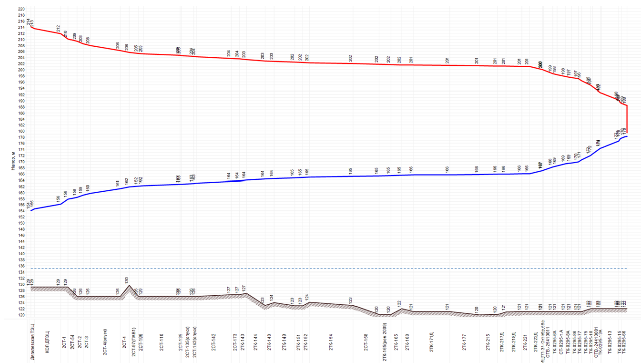
Рисунок 3.13 - Пьезометрический график
